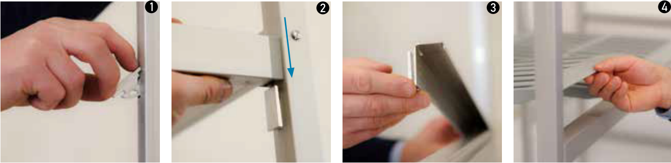
Umiestnite záves do otvoru Zaveste policu Zaveste rohový úchyt Umiestnite výplne police
